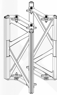
Straight module
